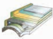
Na klenbách pod betonovou plovoucí podlahou s dodatečnou tepelnou izolací a s uložením rozvodů sítí
