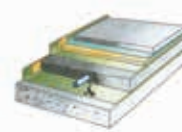
Na betonovém stropě pod betonovou plovoucí podlahou s dodatečnou tepelnou izolací a s uložením rozvodů sítí
